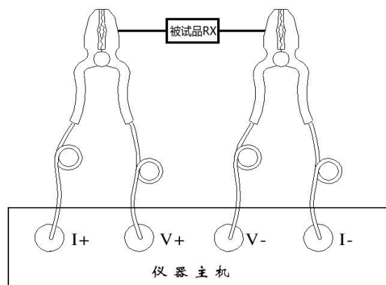
图二 接线图
